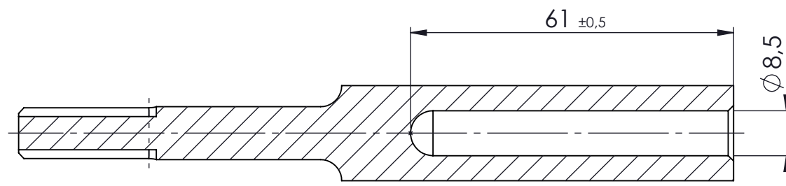
DOORSNEDE A-A
