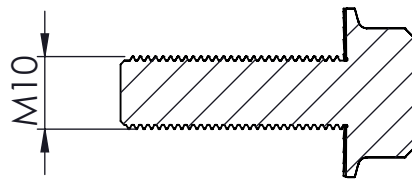
DOORSNEDE A-A
