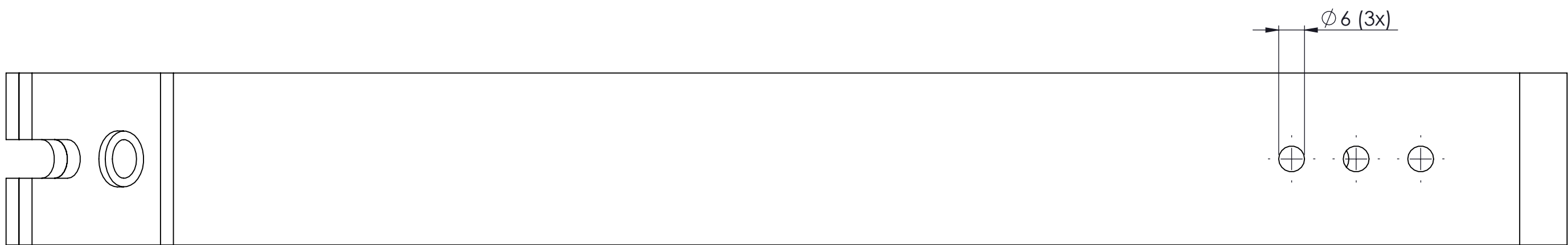
AANZICHT A
